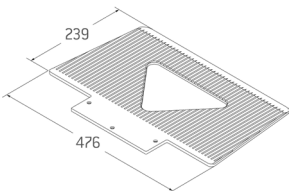
Schaufel GS
