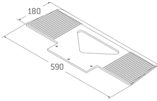
Schaufel XL
