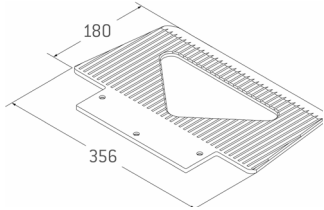
Schaufel L
