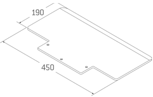
Schaufel DS-NG
