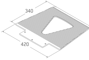
Schaufel G
