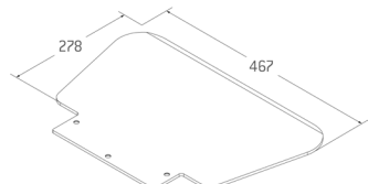
Schaufel LH
